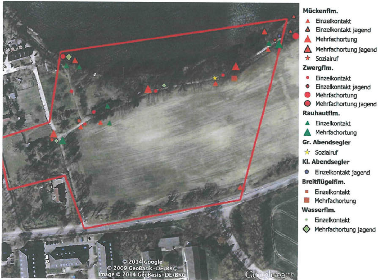
Abbildung 5: Fledermauskontakte im Untersuchungsgebiet Süduferpark (Luftbild aus Google-Earth™)
