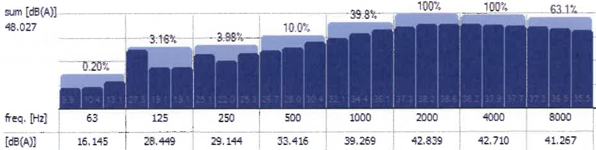
Abbildung 2: Quellenspektrum zur Schallberechnung
