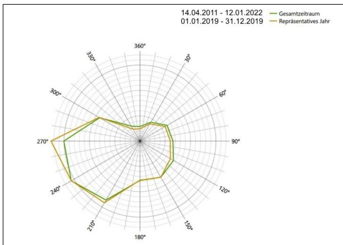
Abbildung 8: Windverteilung Station Dörnick
