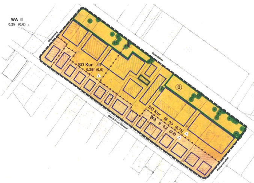
Bild 3: Auszug aus dem Bebauungsplan Nr. 4, 4. Änderung, gültig seit dem 22.01.2003
