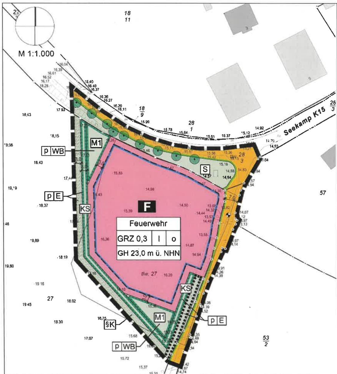
Abbildung 4: Ausschnitt aus dem B-Plan 109, Prokom, 03.06.2024
